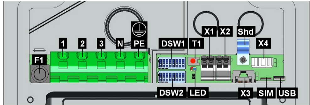
Abb. 7-15: Anschlussübersicht
