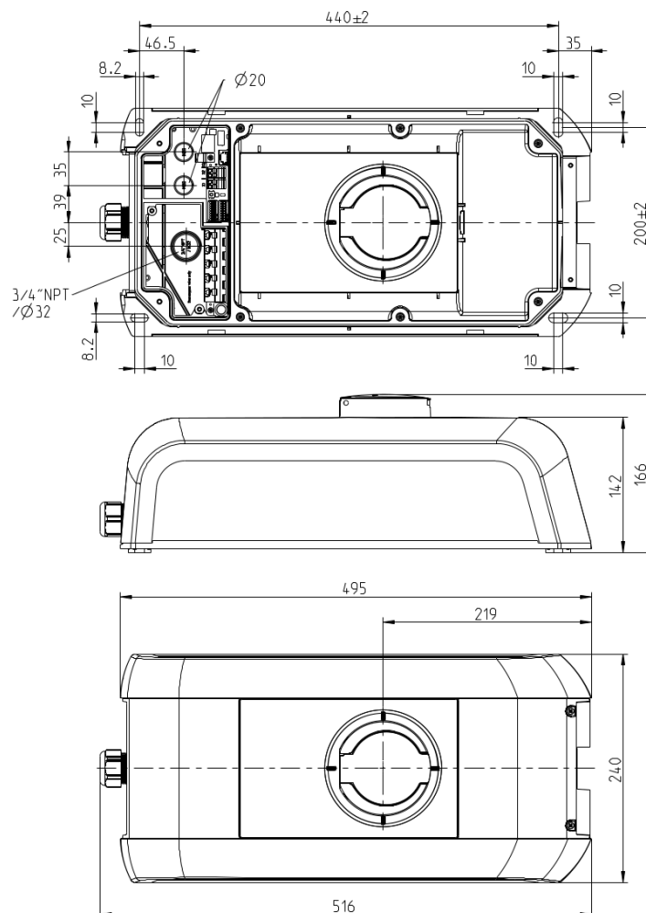
Abb. 12-20: Abmessungen in Millimeter
