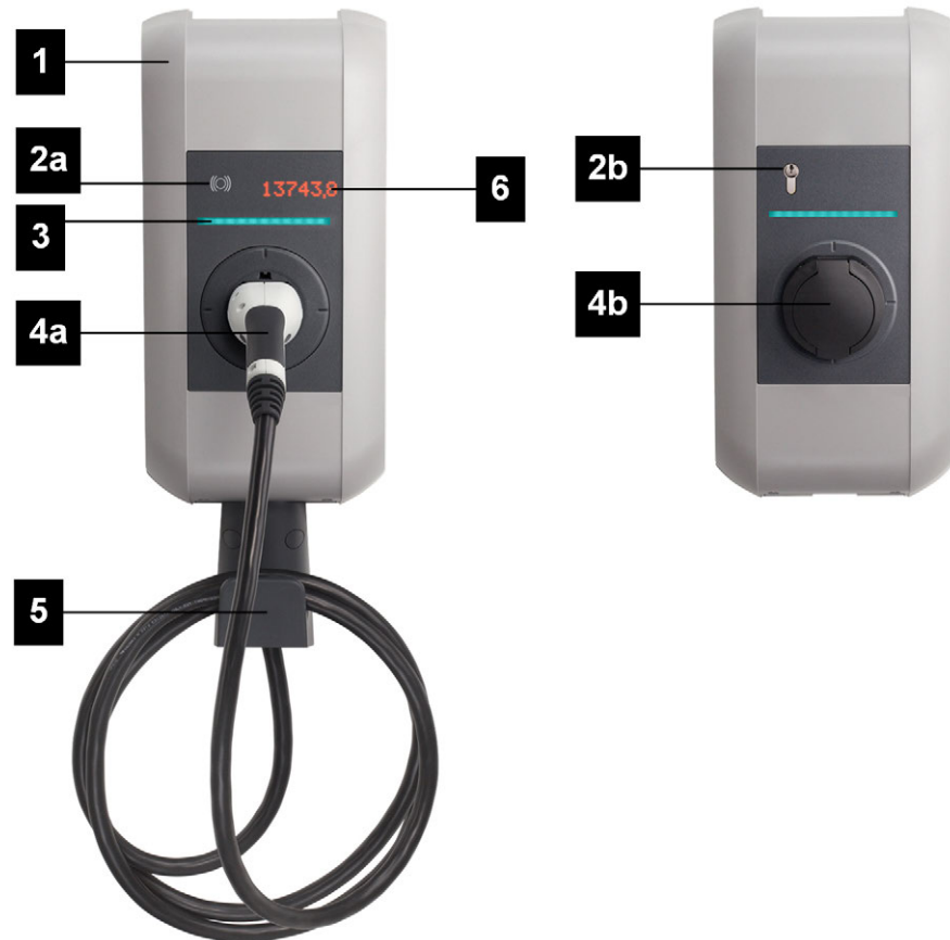
Abb. 4-4: Übersicht Ladestation
