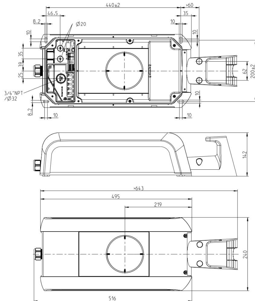
Abb. 12-21: Abmessungen in Millimeter
