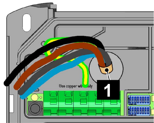
Doppelmembranstutzen (Unterputz Kabelmontage)
