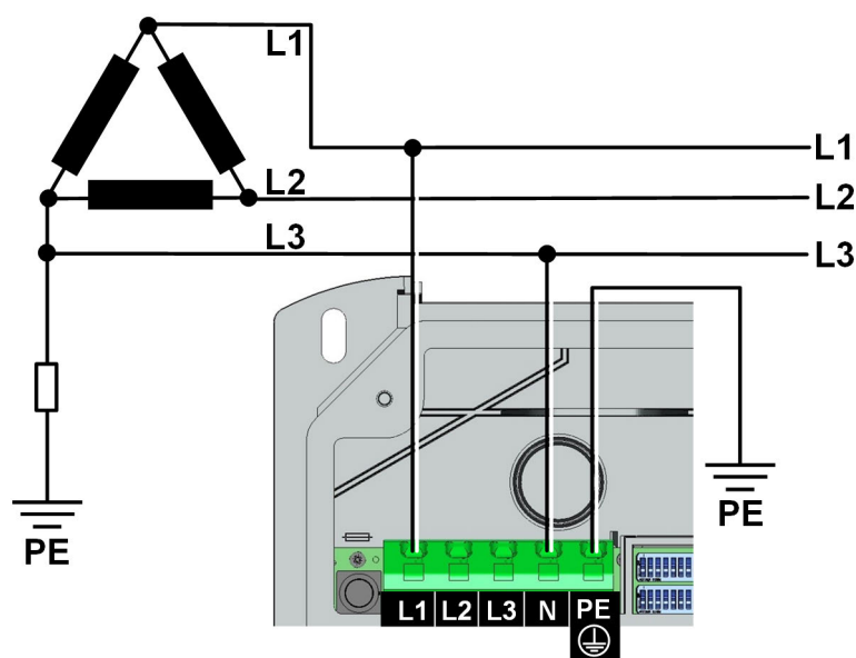
Abb. 7-16: Anschluss an ein Dreileiter-IT-System mit 230 V
