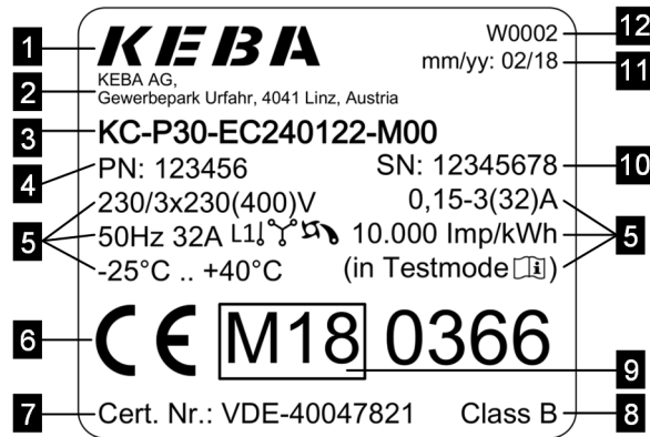
Abb. 3-2: Typenschild (Beispiel)
